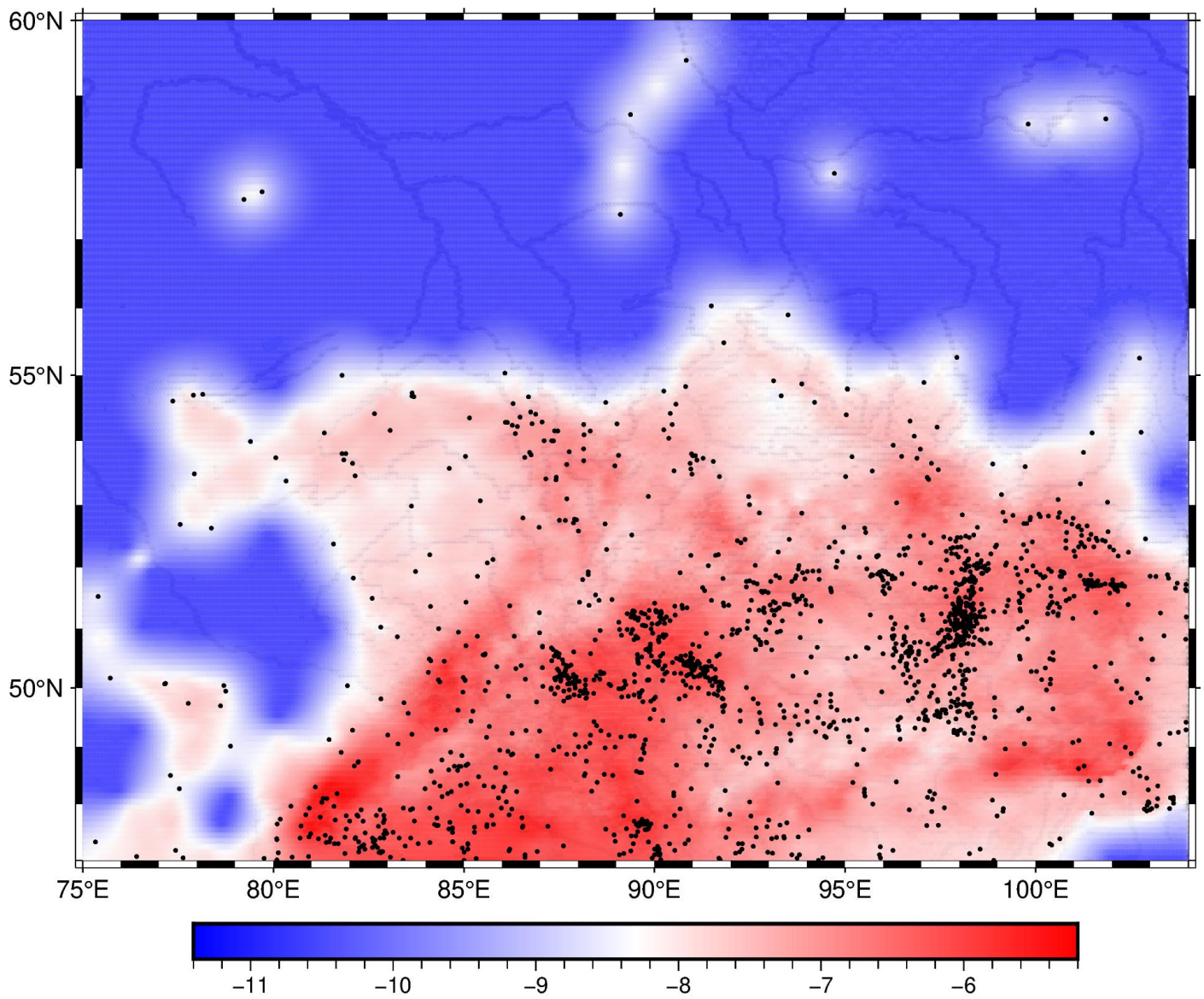
Рисунок 1. Пространственные вариации сейсмической активности для региона Алтай-Саяны a = \log_{10} v , v – оценка числа землетрясений с магнитудой M \geq 8.0 в ячейке 0.1^\circ \times 0.1^\circ в год. Землетрясения показаны точками. Значения a присваивались геометрическому центру эпицентров землетрясений, попавших в круг сканирования радиуса R = 100 км.
