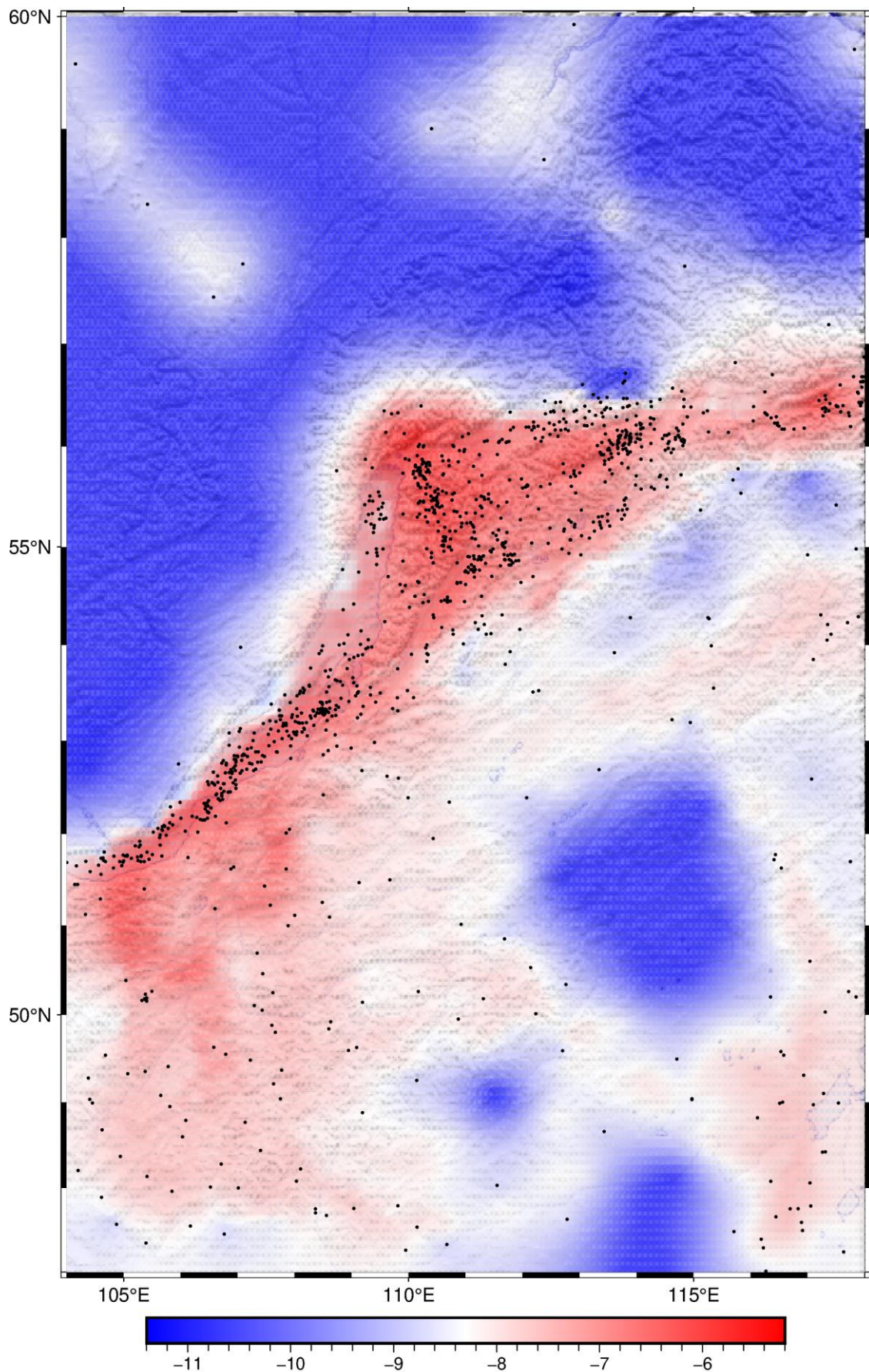
Рисунок 1. Пространственные вариации сейсмической активности для региона Прибайкалье a = \log_{10}v , v – оценка числа землетрясений с магнитудой M \geq 8.0 в ячейке 0.1^\circ \times 0.1^\circ в год. Землетрясения показаны точками. Значения a присваивались геометрическому центру эпицентров землетрясений, попавших в круг сканирования радиуса R = 100 км.
